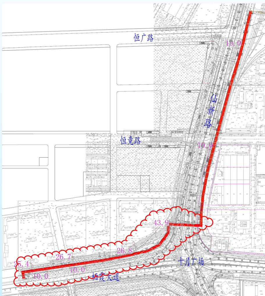
仙新路段管廊平面图 - 变更前
