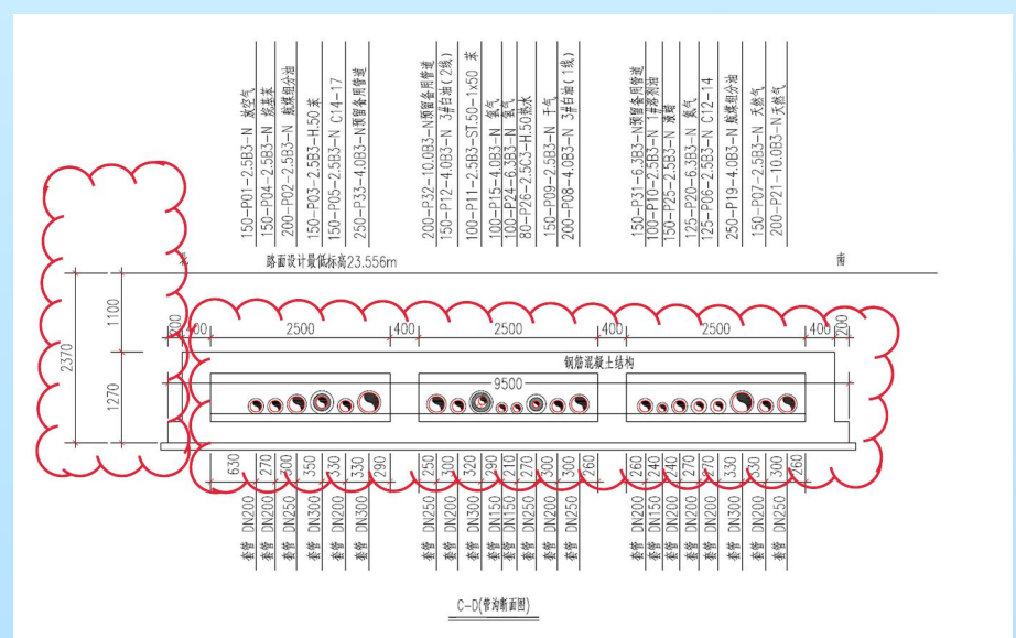
仙新路段管沟剖面图 - 变更后
