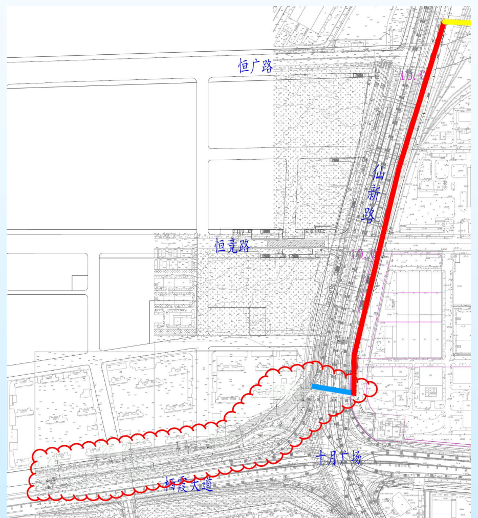
仙新路段管廊平面图 - 变更后
