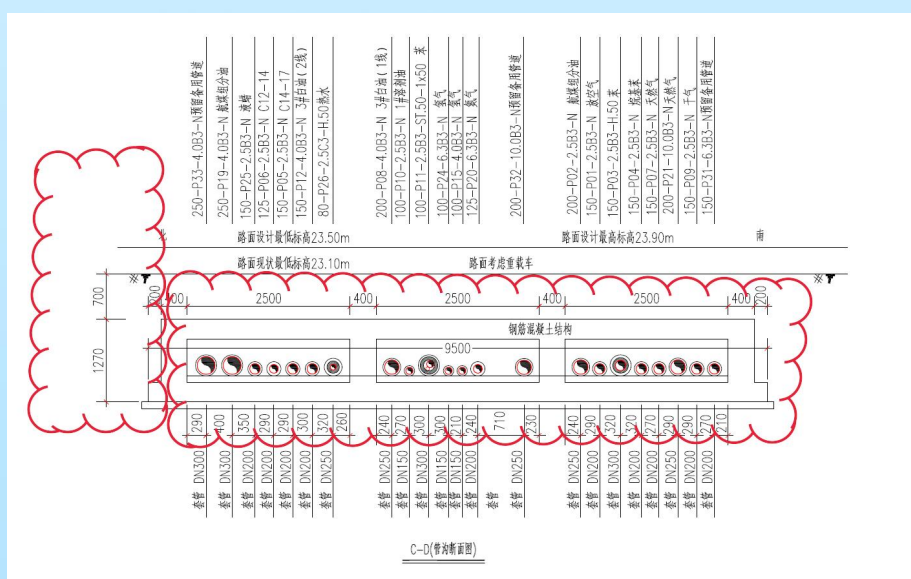
仙新路段管沟剖面图 - 变更前
